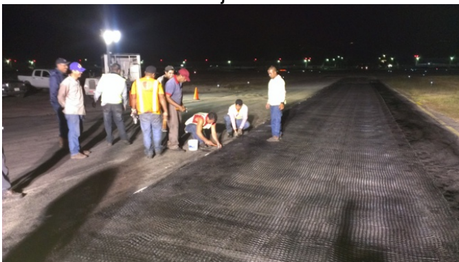
Instalación de Geomalla
